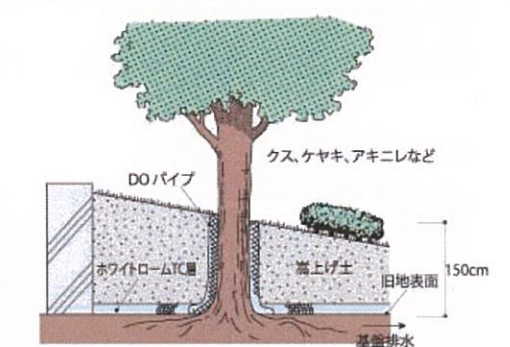
樹木周辺嵩上げ工事断面図
