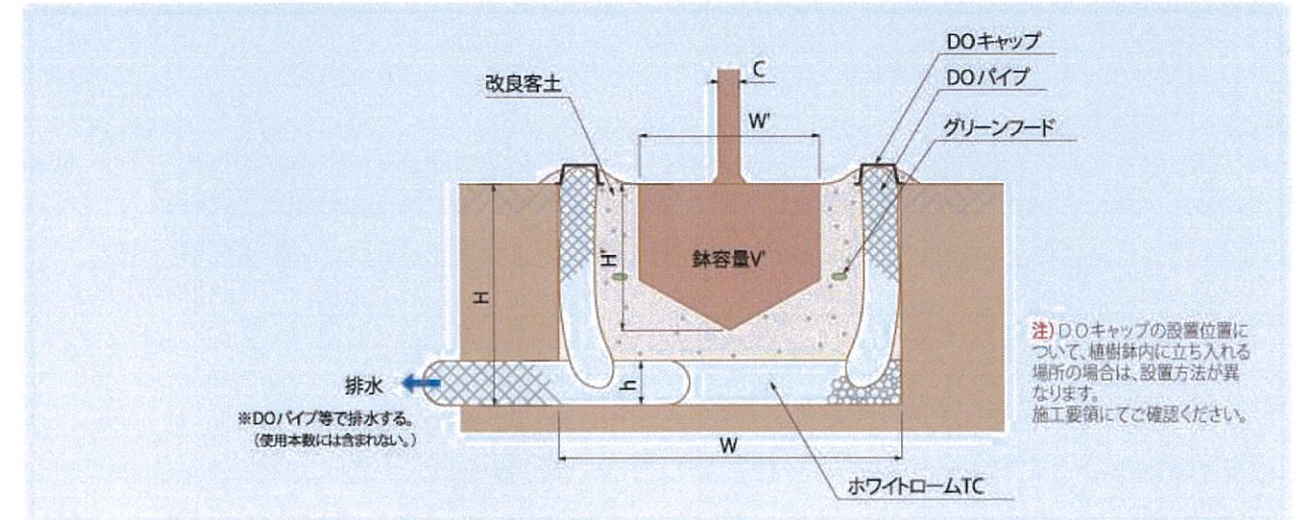
植穴改良表(粘質土の場合)
