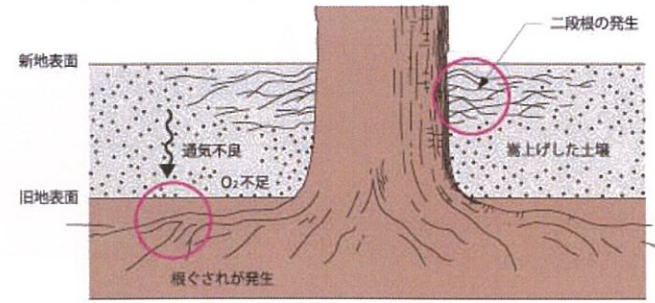
図1：樹木周辺嵩上げによる二段根の発生図
