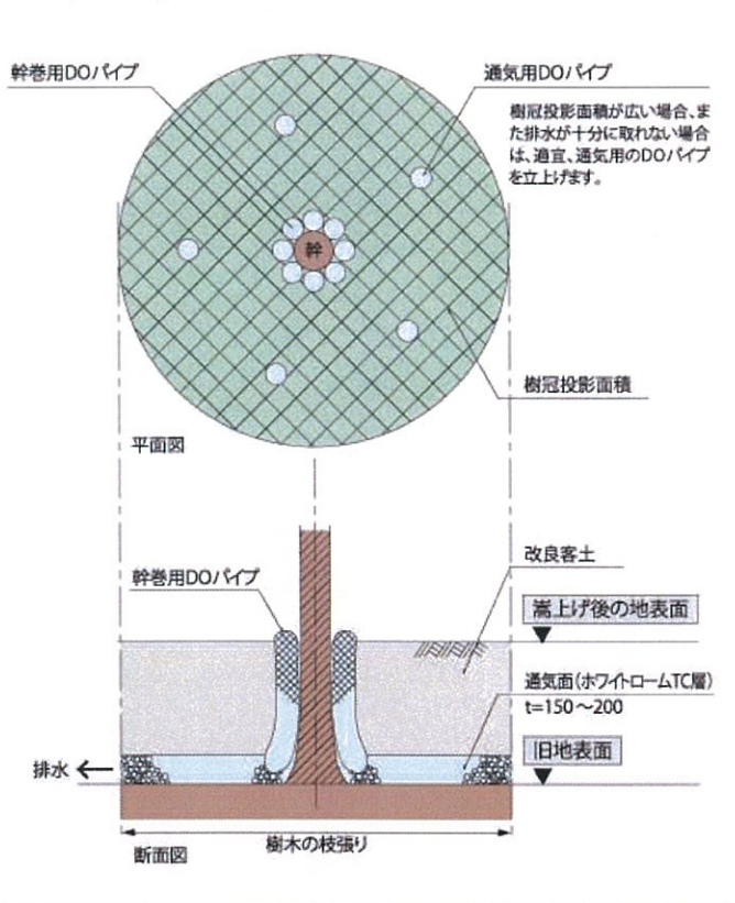
図2：既存樹木の周辺嵩上げ対策 標準図
